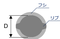
異形丸鋼
